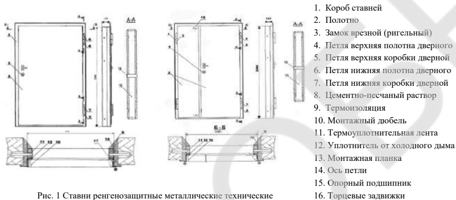
Рис. 1 Ставни рентгенозащитные металлические технические
